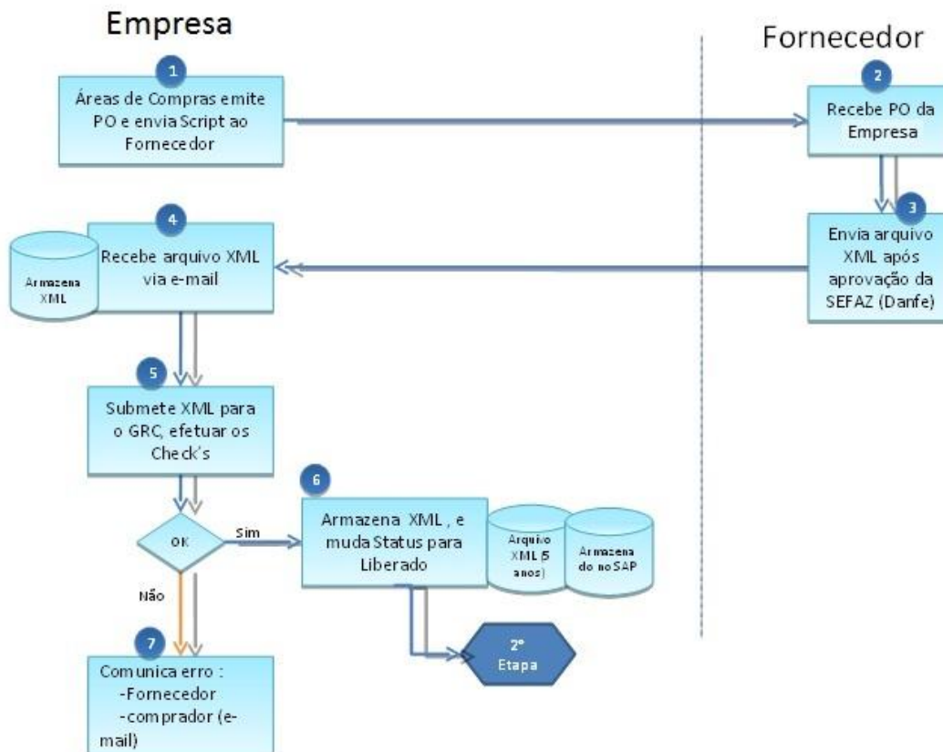
Figura 4: Etapa 1 – Fluxo do Recebimento/Verificação interna da consistência e leiaute/schema do XML.
