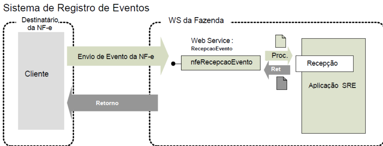
Figura 2: Serviço destinado à recepção de mensagem de Evento da NF-e.
